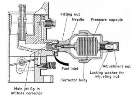
Fig. 41 SOLEX Altitude Corrector
